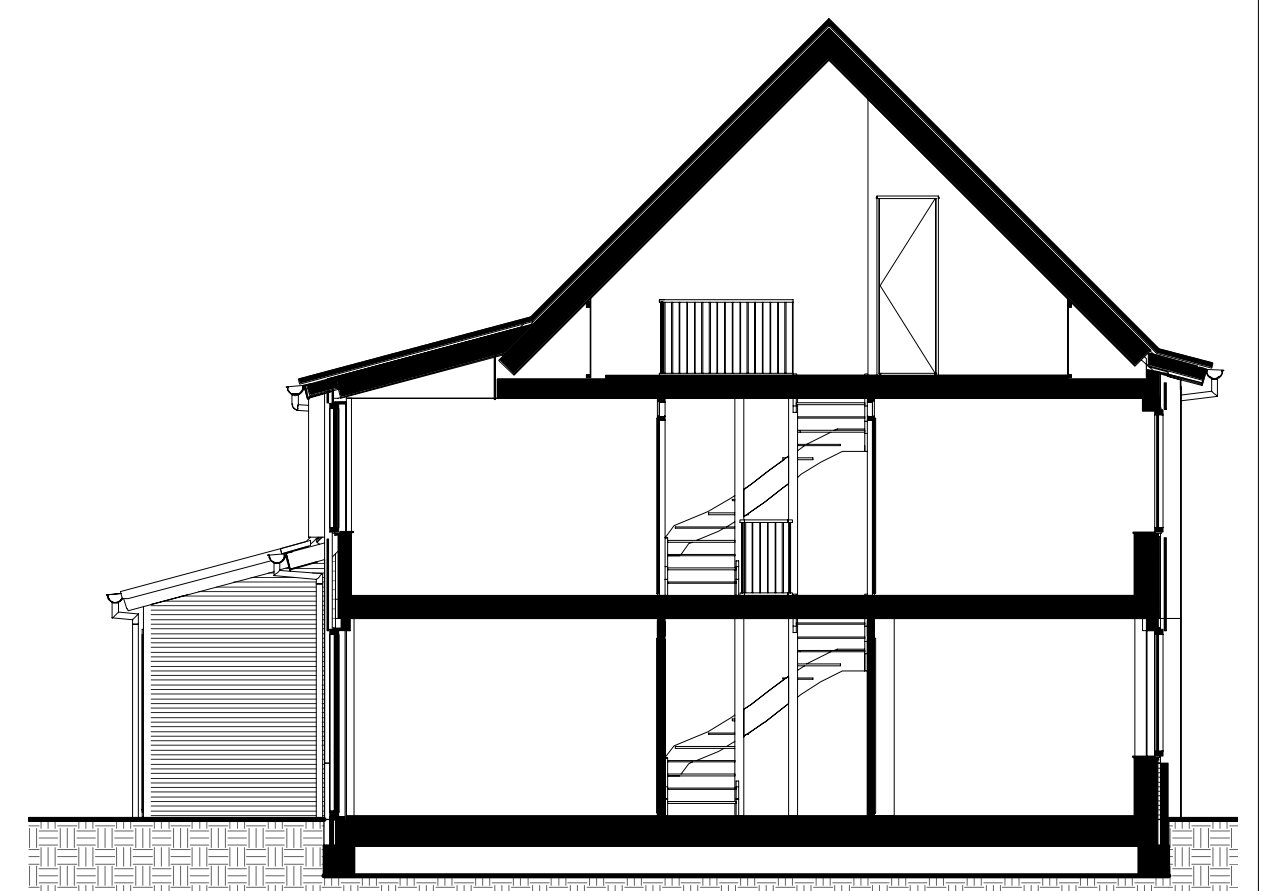
doorsnede A-A, Blok 16
