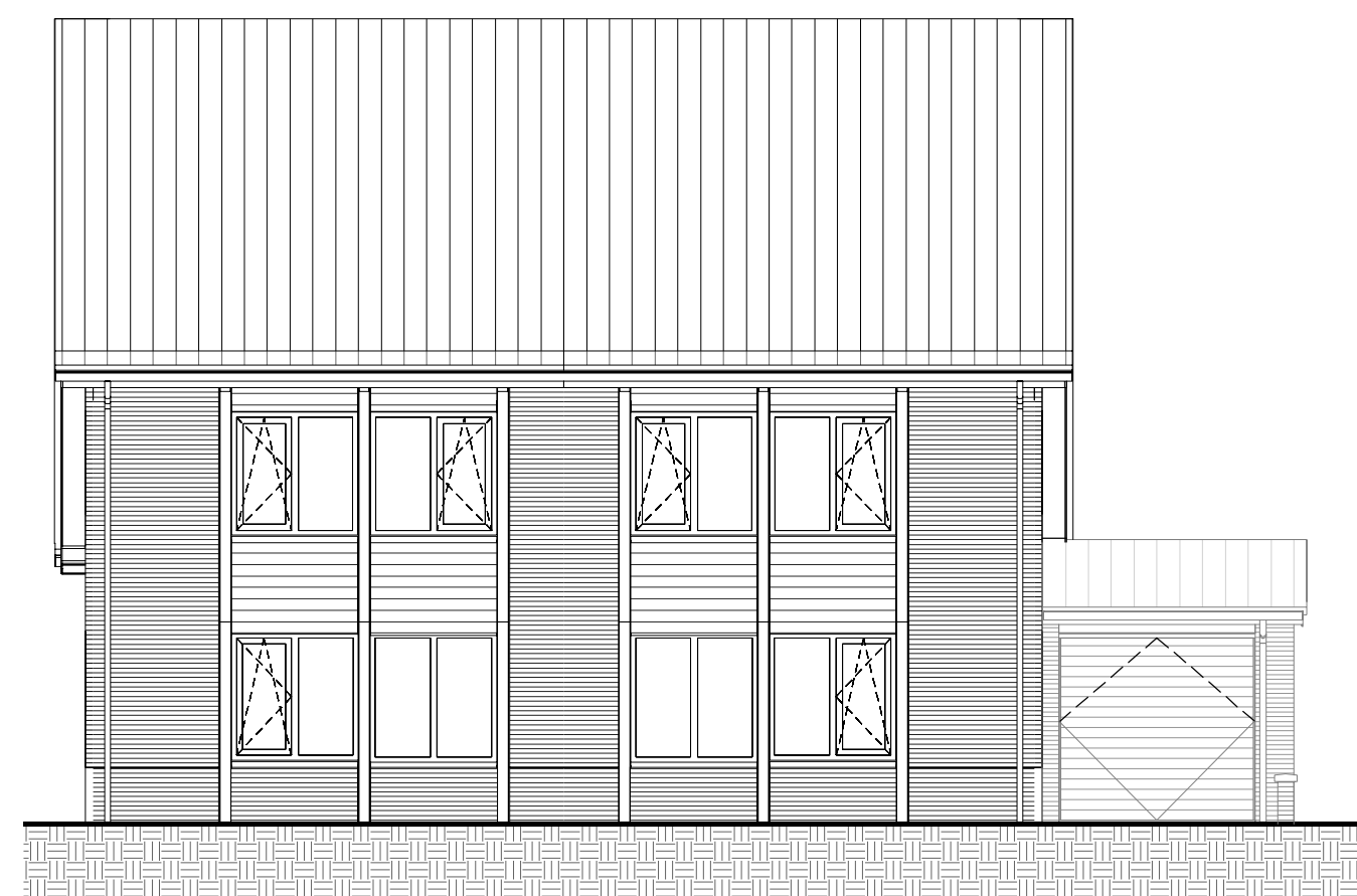
voorgevel
