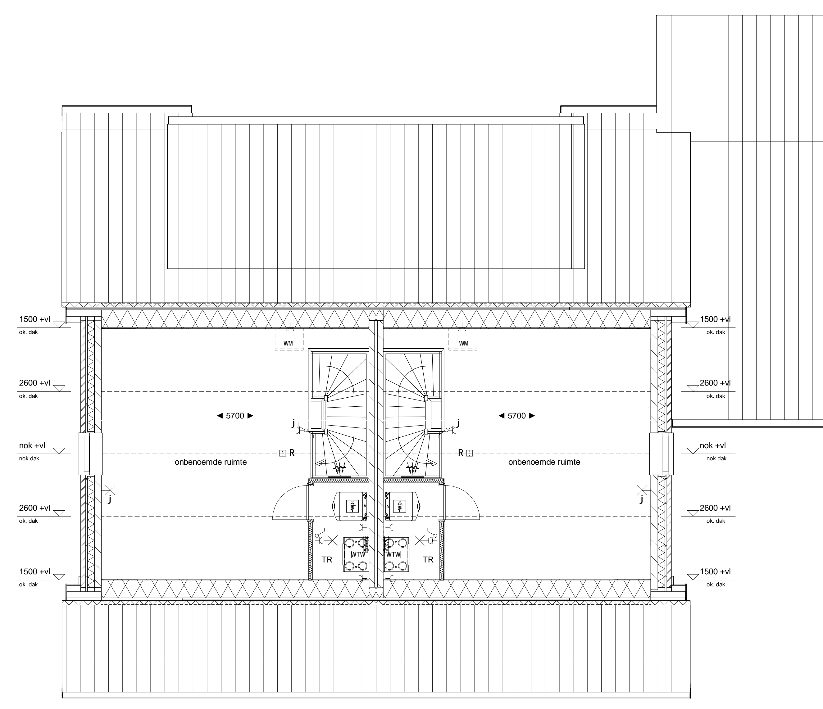
2e verdieping
