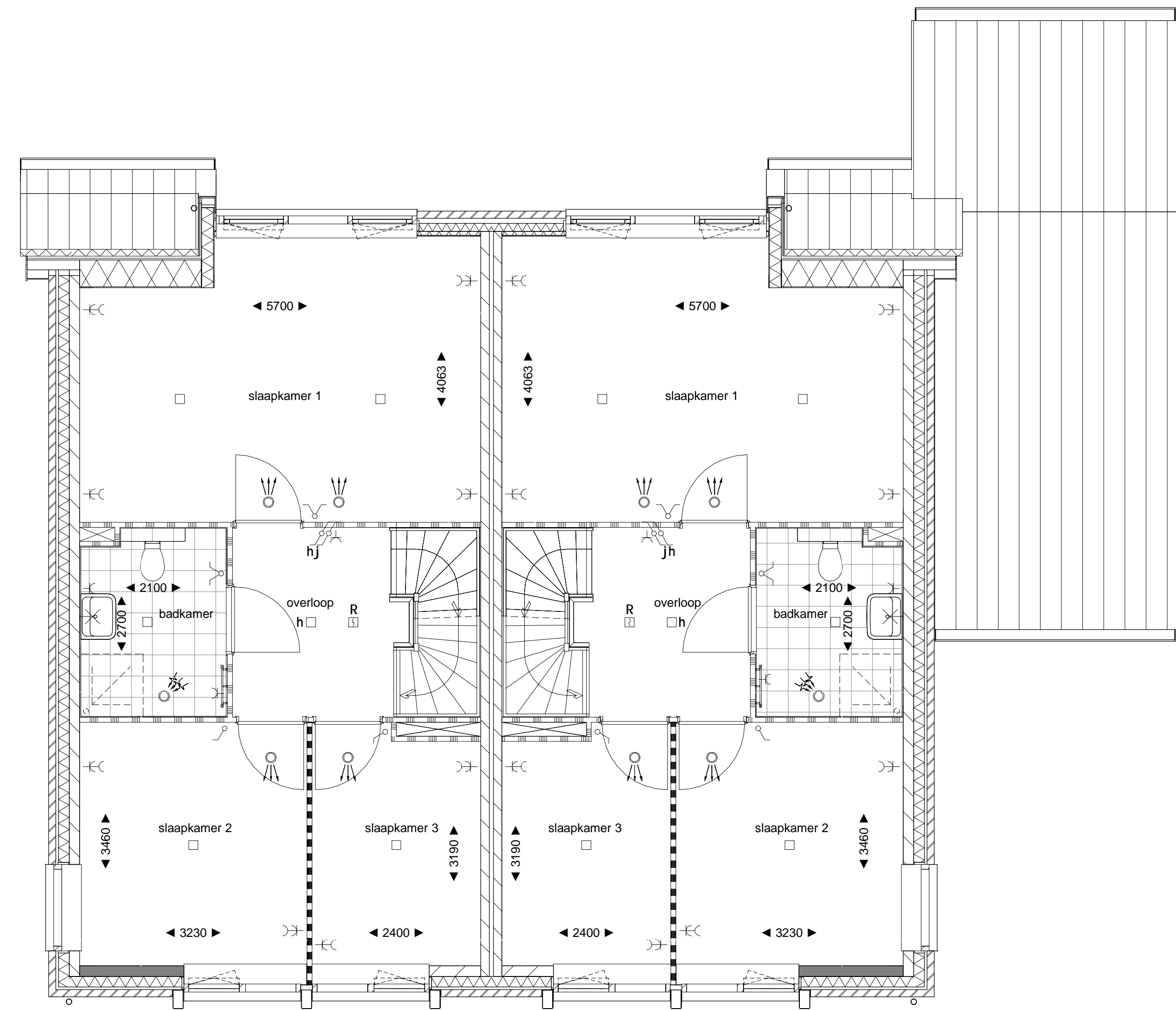
1e verdieping
