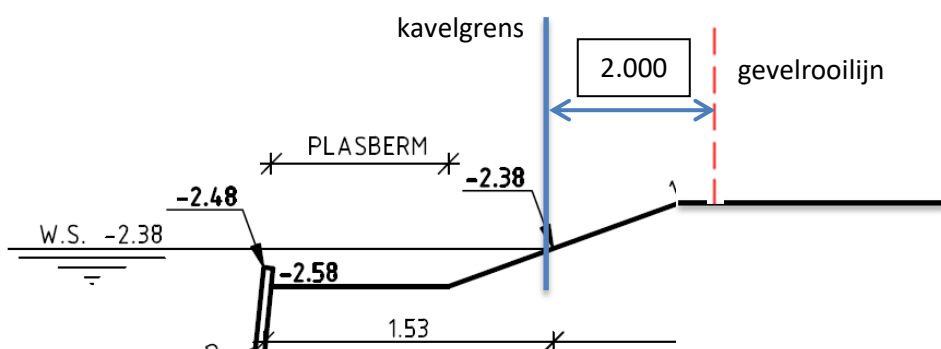
Doorsnede t.p.v. plasberm (oostelijke zijde van de kavel)
